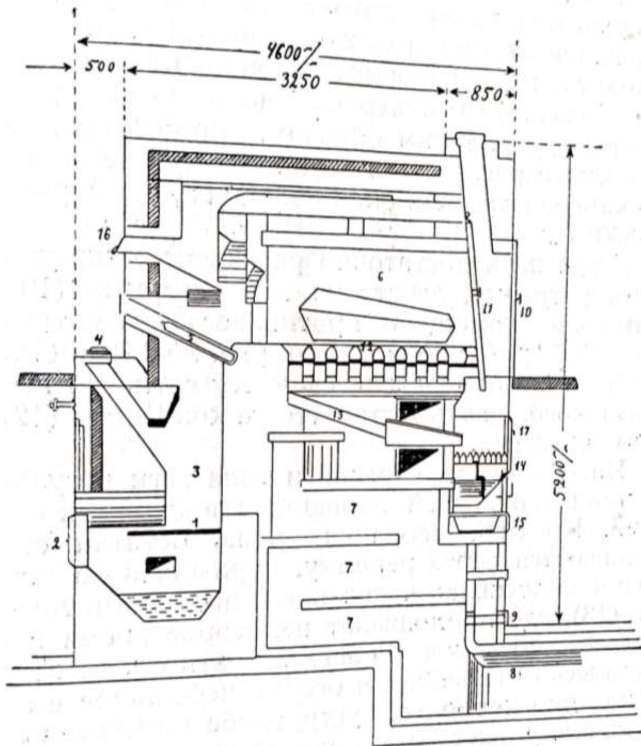
Рис.9. Продольный разрез кремационной немецкой печи фирмы Топф.
