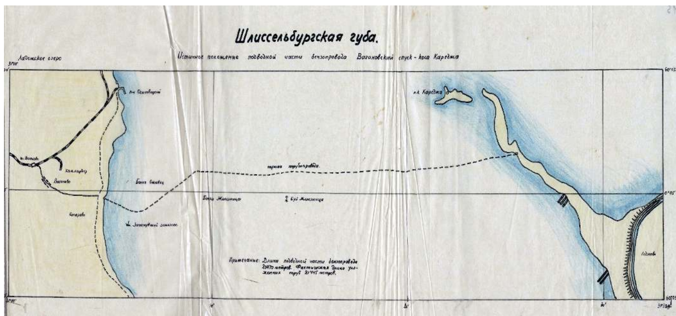
Рис. 10. Маршрут прокладки трубопровода по дну Ладожского озера.
