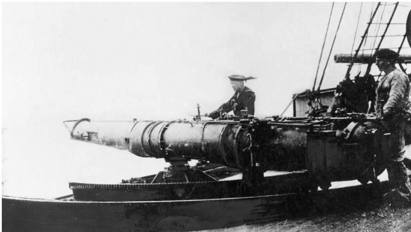
Рис.7. Торпедный аппарат.
