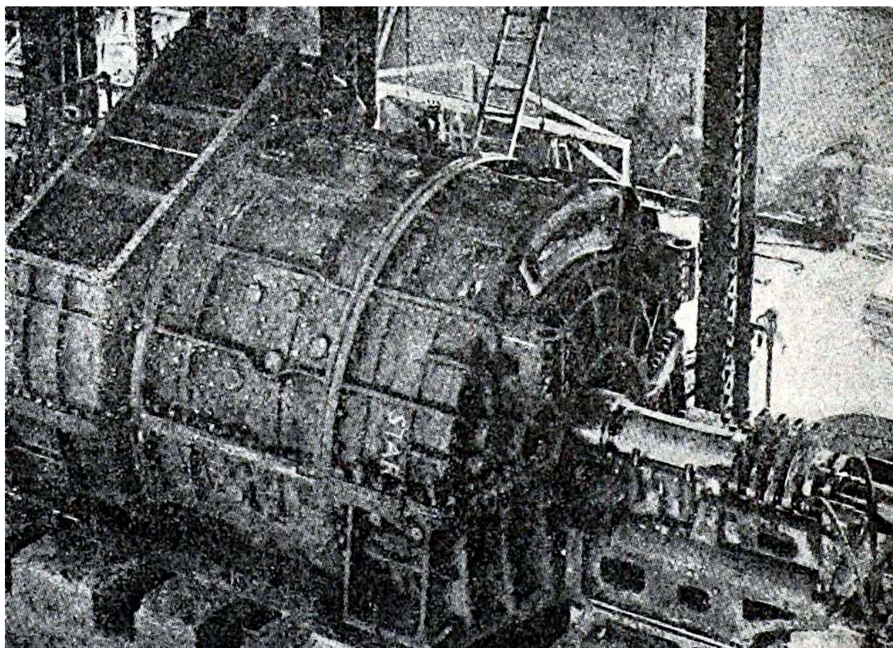
Рис.6. Судовая турбина.
