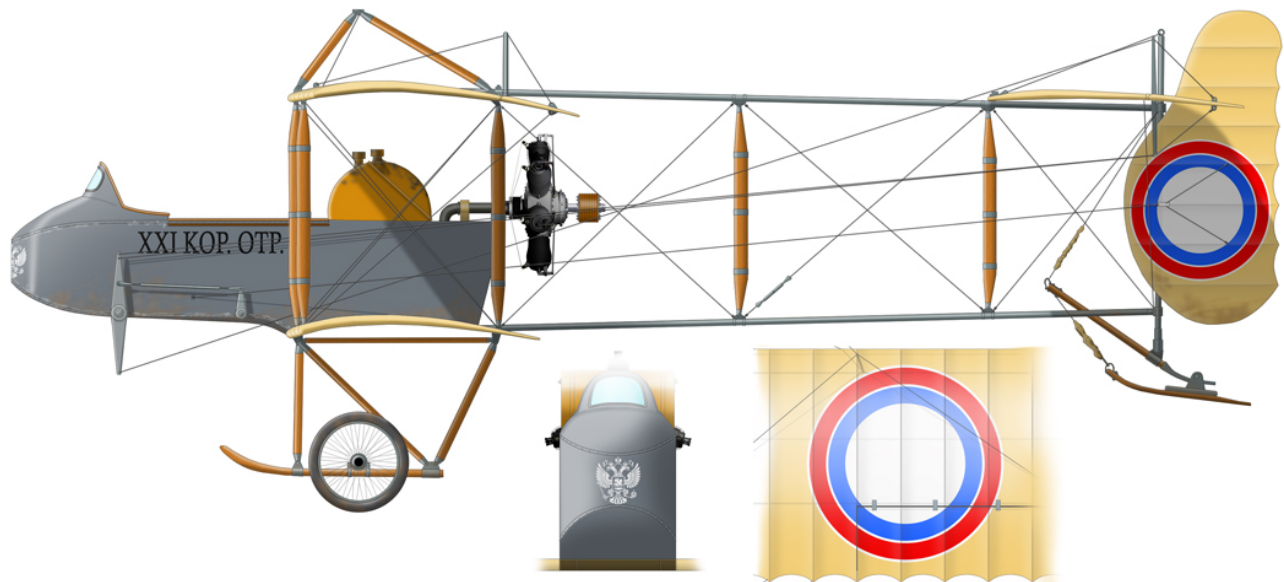
Рис. 2. Русский аэроплан фарман.
